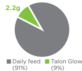
Talon Glow Rats (LD50)
