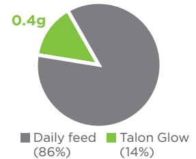
Talon Glow Mice (LD50)
